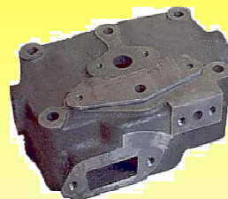
C534 CABEZA COMPRESOR MIDLAND GDE. 2 3/4 JAMSA
