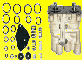
172 RPTO.VAVL.DOBLE MV-2 C/RESORTES BENDIX
