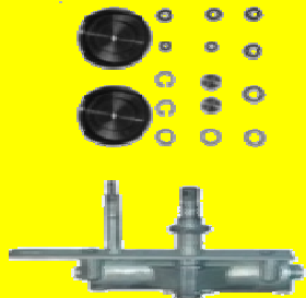
382 RPTO.P/MOTOR LIMPIABRISAS T/CPV AM1081 4" BRAS.
