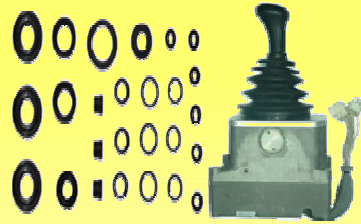
753 RPTO.PALANCA D CAMBIOS MULTEGO 6038.002.029
