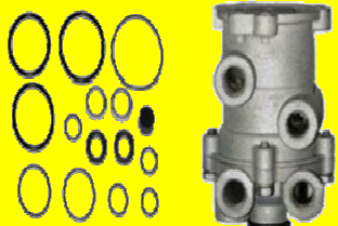
104 RPTO.VALVULA DE PIE E-12 MENOR
